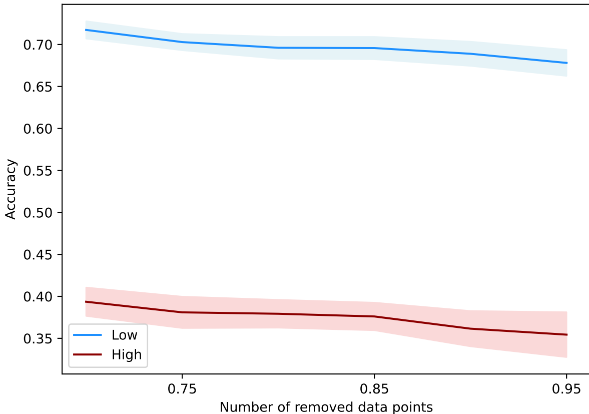
DataAttrOpt(10000, 0.03, 15, inf, +b, alpha=1.0) - adult
